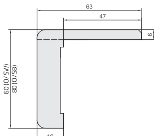
Rohový prvok zárubne SW predĺžená obložka o 2 cm
