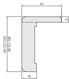
Rohový prvok zárubne SW obložka standard
