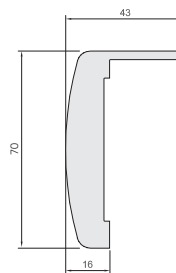
Rohový prvok zárubne LUX obložka standard
