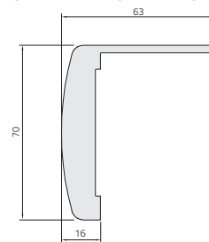
Rohový prvok zárubne LUX predĺžená obložka o 2 cm
