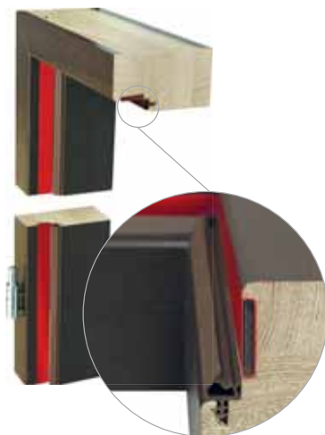
klesajúce tesnenie naspodu kridla (verzia 2)
