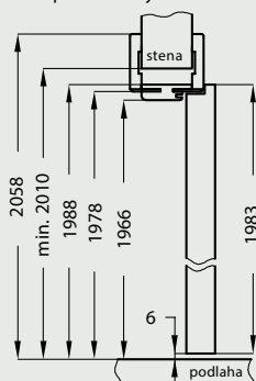
Zvislý prie rez poldrážkových dverí
