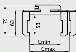
Prie rez OR
